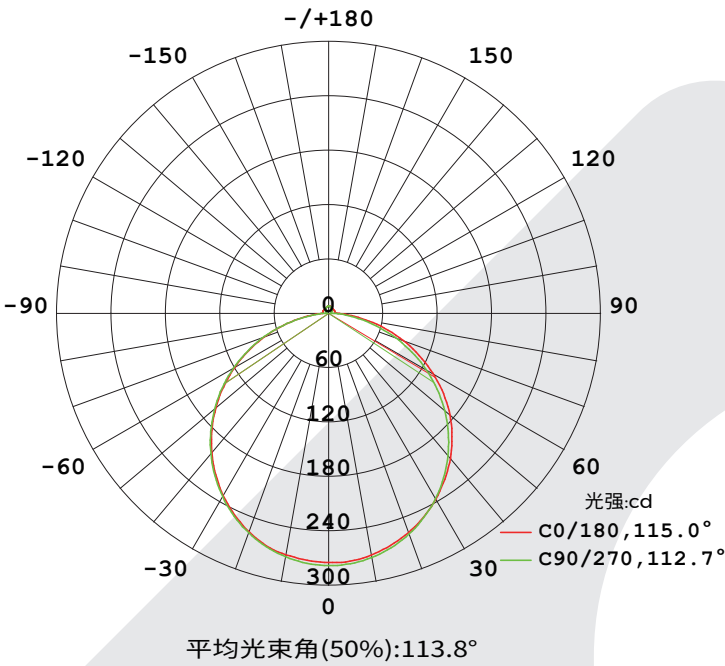
配光曲线
